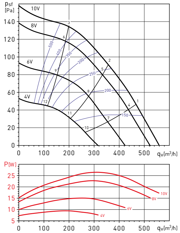
CTB-500/200 ECOWATT
