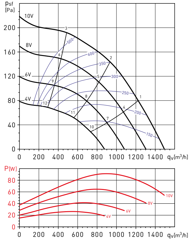
CTB/4-1300/315 ECOWATT
