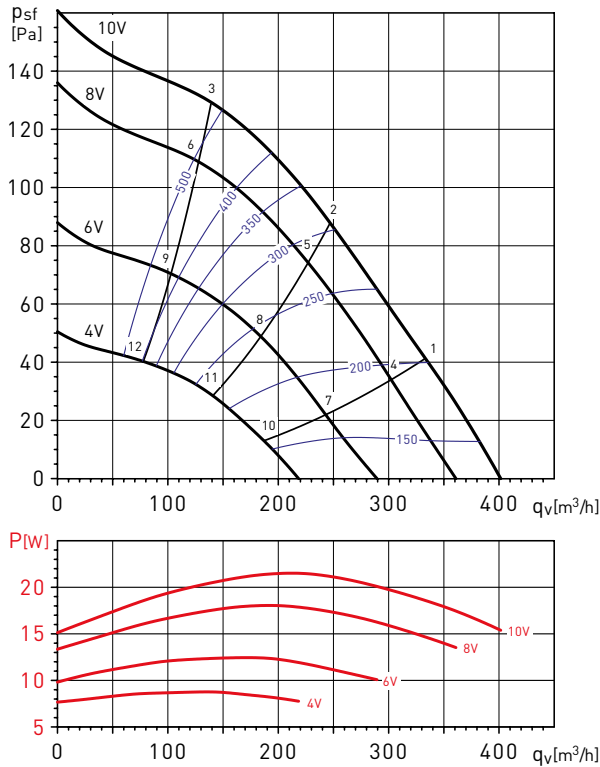
CTB-400/160 ECOWATT
